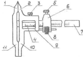
Рис.3. Штангенциркуль ШЦ-2.
