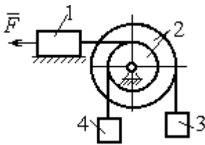
Рис. 6.30. Схема подъёмника
