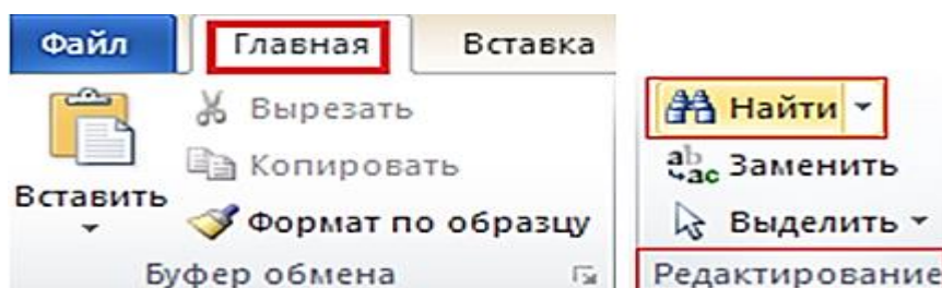
Рис. 31. Область навигации
