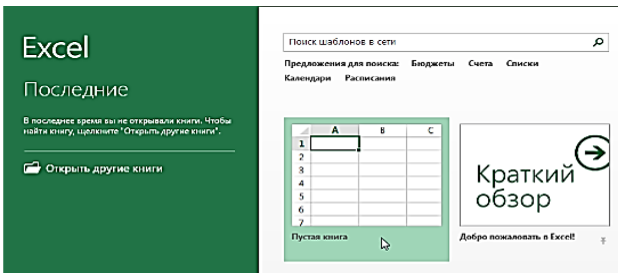
Рис. 1. Начальный экран
