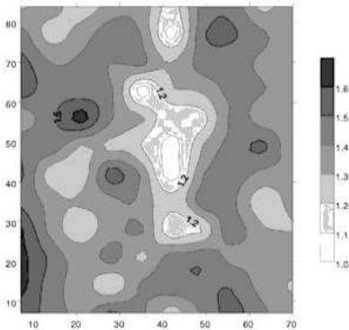
Рис. XX.6. Поверхность, отражающая пространственное варьирование плотности серых лесных почв Владимирского опоя в июле 1996 года на глубине 35–40 см. Метод построения – метод кригинга (Kriging), для аппроксимации семивариограммы использовалась линейная модель с нулевым паттерн-эффектом
