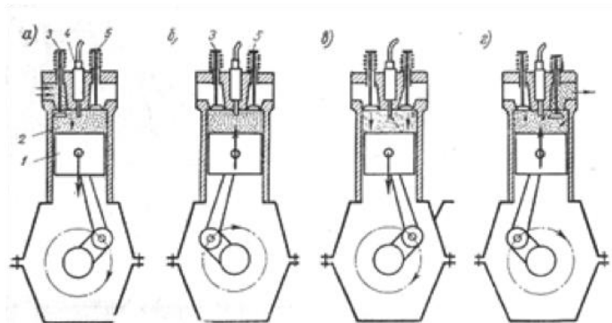
Рис.1. Рабочий процесс четырехтактного двигателя
