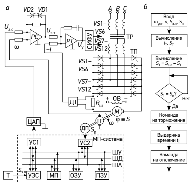
Рис. 6.2. Электропривод с микропроцессорным управлением:
