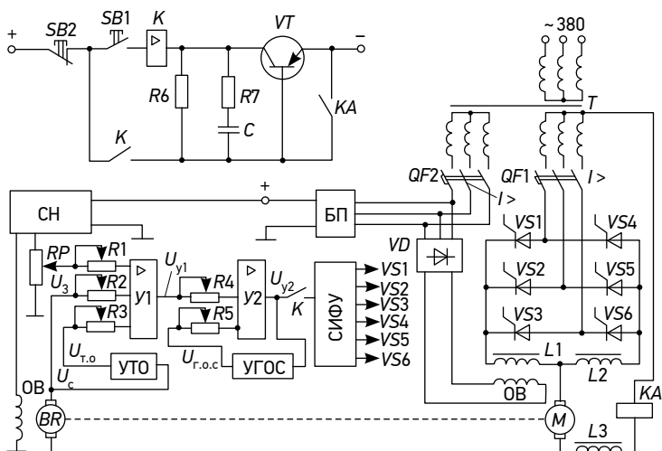
Рис. 6.1. Схема серийного электропривода типа ЭТЗР
