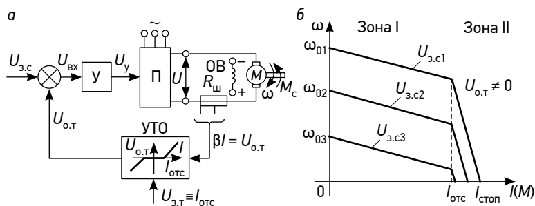
Рис. 4.2. Замкнутая система с обратной связью по току:
