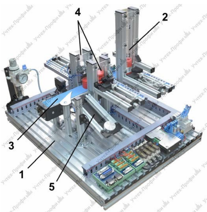
Рисунок 4 – Мехатронный модуль – сборка деталей
