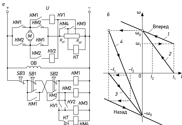
Рис. 3.3. Схема управления: а — пуском и реверсом двигателя, б — характеристики двигателя
