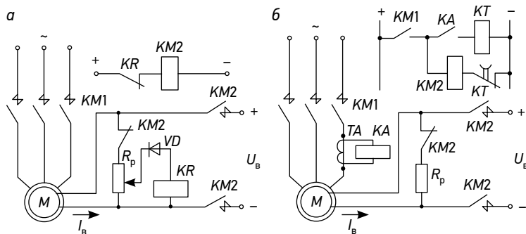
Рис. 9.4. Узлы схем управления возбуждением синхронного двигателя: а — с использованием принципа скорости, б — тока
