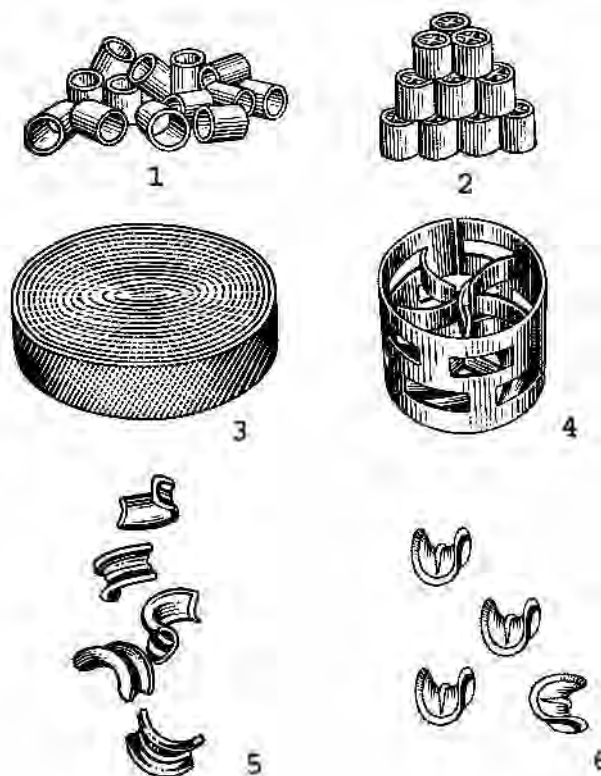
Рисунок 5.1. Типы насадок применяемых в насадочных абсорберах; 1 - кольца Рашига обычные; 2- кольца Рашига с перегородками; 3- насадка Гудлос; 4 - кольца Паля; 5 - насадка "Инталлокс"; 6 - насадка Берля.
