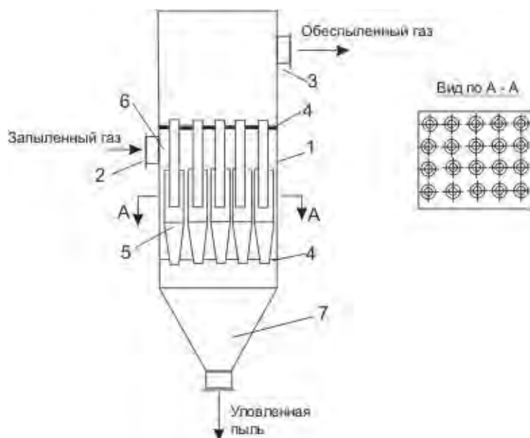
Рисунок 2.2. Батарейный циклон:
