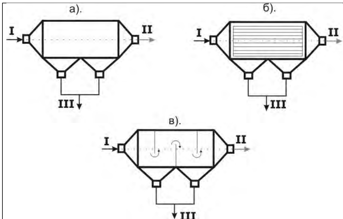
Рисунок 1 Пылеосадительные камеры:
