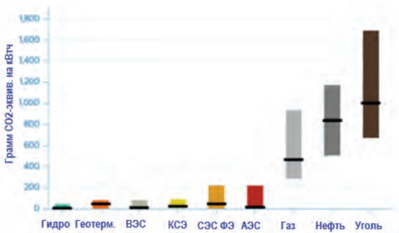
Рис. 15. Эмиссии жизненного цикла различных технологий
