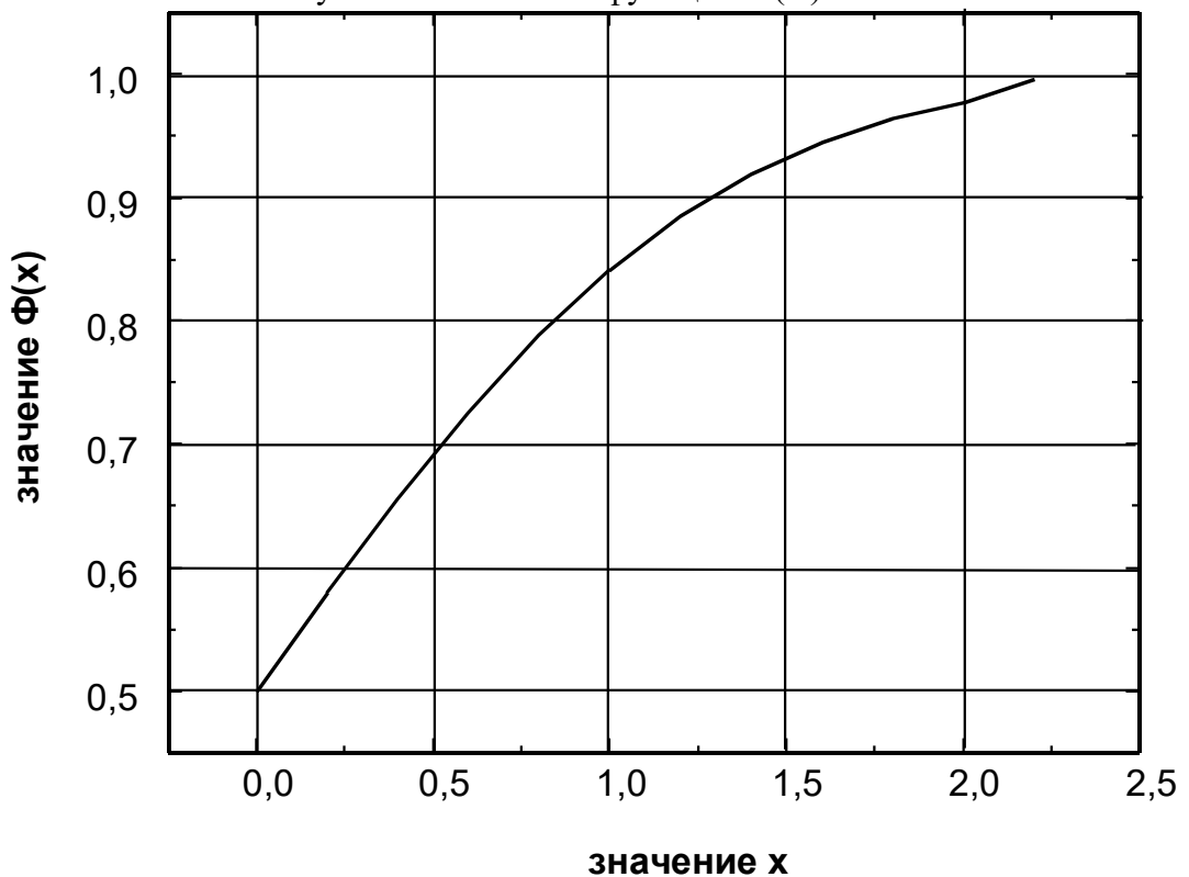
Рисунок 2.5. Значение функции \Phi(X) .
