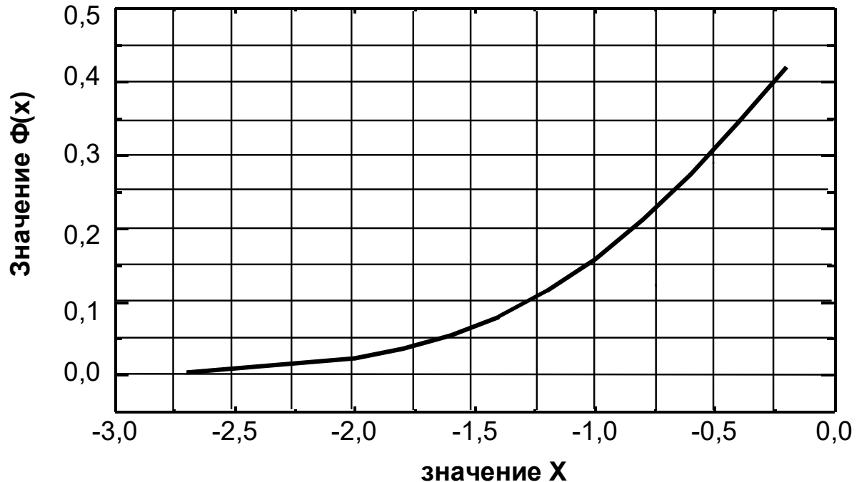
Рисунок 2.4. Значение функции \Phi(X)
