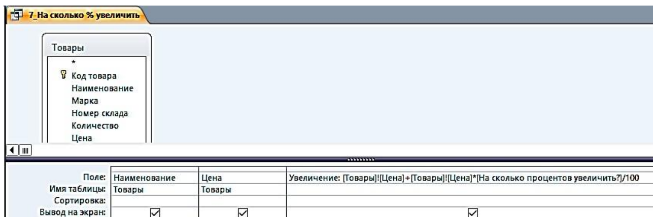
Рис. 2.13. Использование параметра в выражении вычисляемого поля
