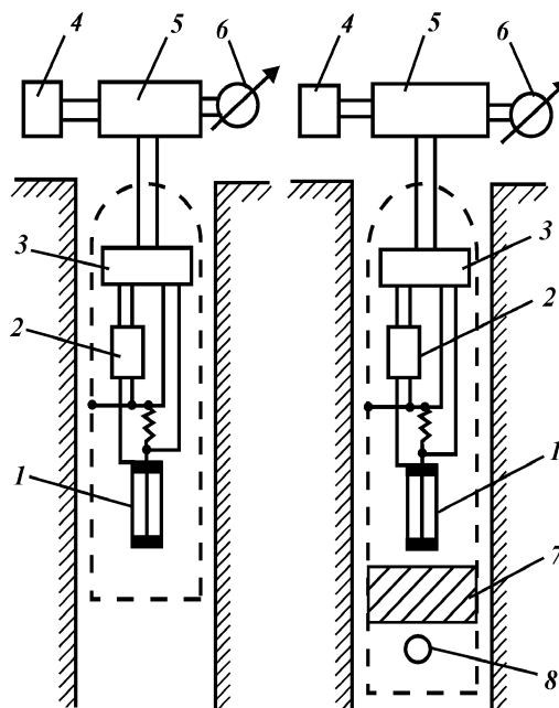
Рис. 1.1 Принципиальные схемы измерений гамма-метода (а) и IАЕ-тронового гамма-метода (б):
