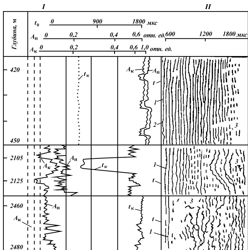
Рис. 1.7. Совместная регистрация цементограммы (I) и фазокоррелогаммы (II): I – линии первых вступлений акустической волны по колонне A_{\kappa} ; 2, 3 – сдвиги линий волн по колонне A_{\kappa} и породе A_{\pi}
