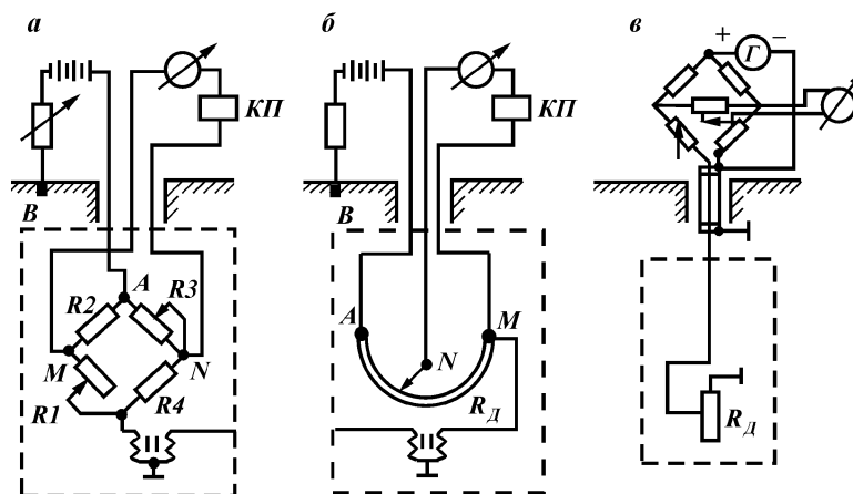
Рис. 1.4. Электрические схемы кавернометров для работы с трех- (а, б) и одножильным (в) кабелями:
