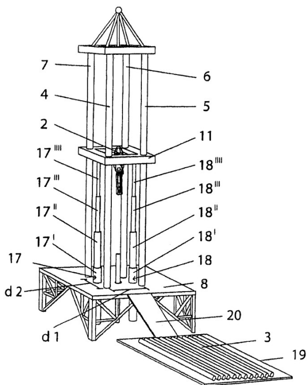
Рисунок 2 – Буровая установка,..... 2
