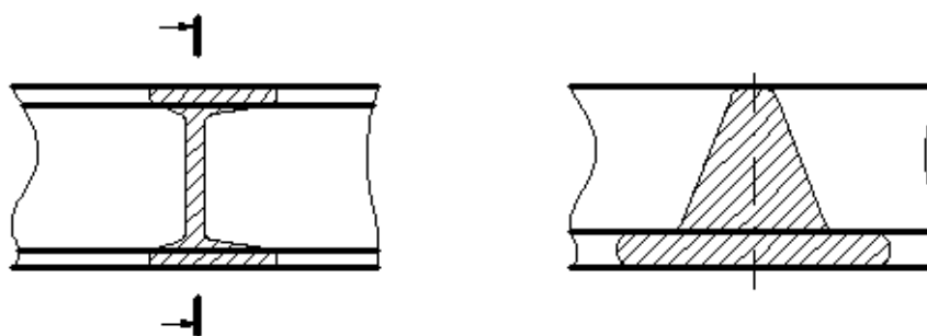
Рис. 25. Наложенные сечения
