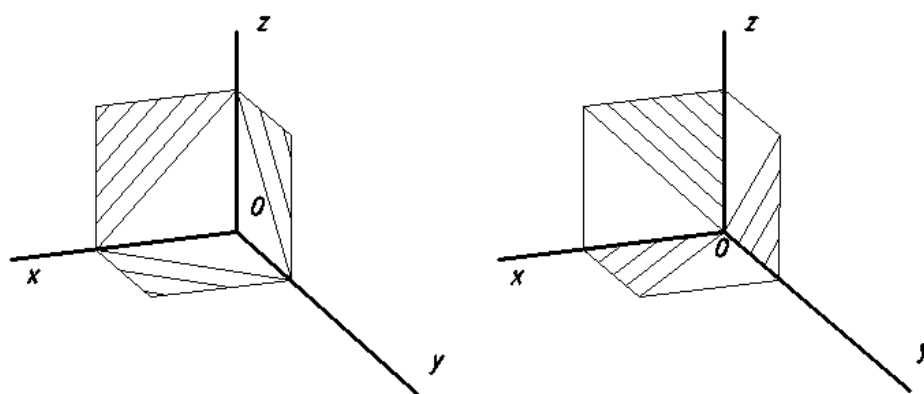
Рис. 42. Нанесение линий штриховки: а) в прямоугольной изометрии; б) в прямоугольной диметрии
