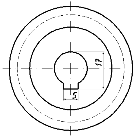
Рис. 36. Группировка размеров, относящихся к одному элементу
