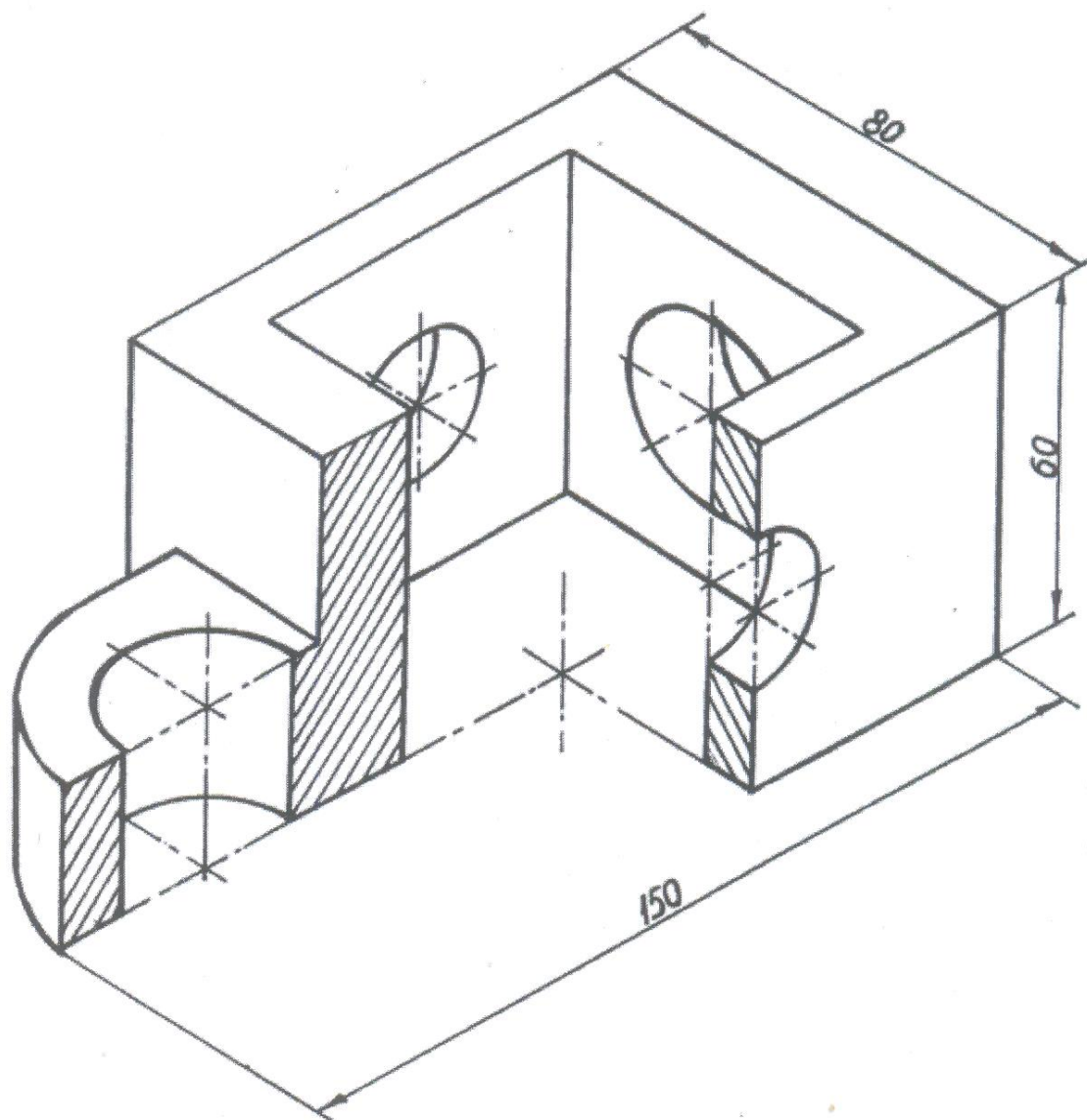
Рис. 40. Изображение детали в прямоугольной изометрии
