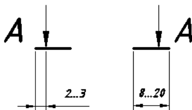
Рис. 18. Обозначение разреза
