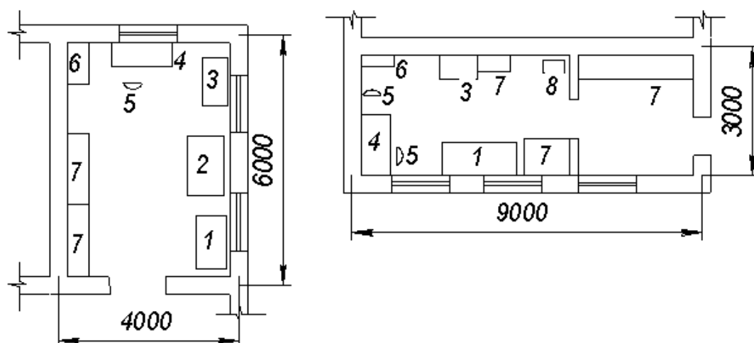
Рисунок 5 – Компоновка постов электрика по типовому (а) и индивидуальному (б) проектам:
