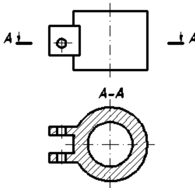
Рис. 13. Горизонтальный разрез
