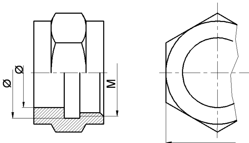
Рис. 28. Нанесение размерных линий с обрывом
