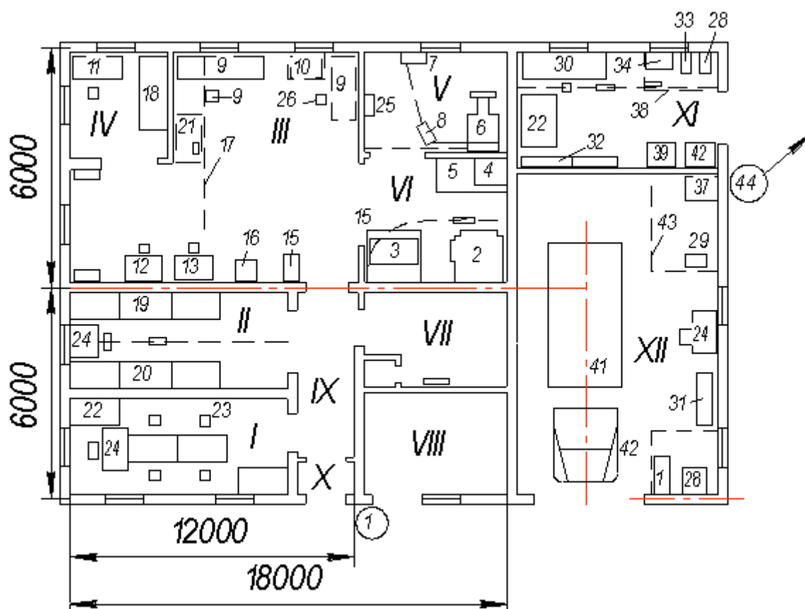
Рисунок 3 – Компоновка пунктов технического обслуживания и ремонта электрооборудования по индивидуальному (а) и типовому (б) проектам:
