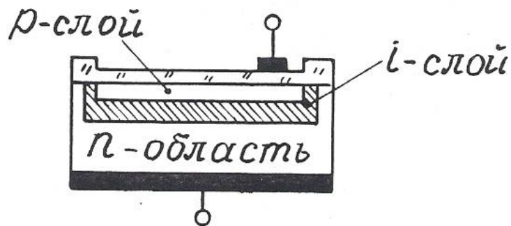
Рис. 3.9. Структура pin-диода
