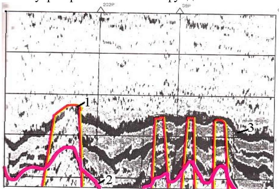
Рис.1.1. Фрагмент временного разреза с субвертикальными зонами деформации (СЗД). Краснелининский свод (западная Сибирь). 1-проявления СЗД; 2- граница фундамента; 3- отражающие горизонты [5]
