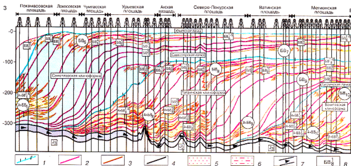
Рис.1.5. Принципиальная схема геологического строения западной части Нижнеартвовского свода (А. Л. Наумов)
