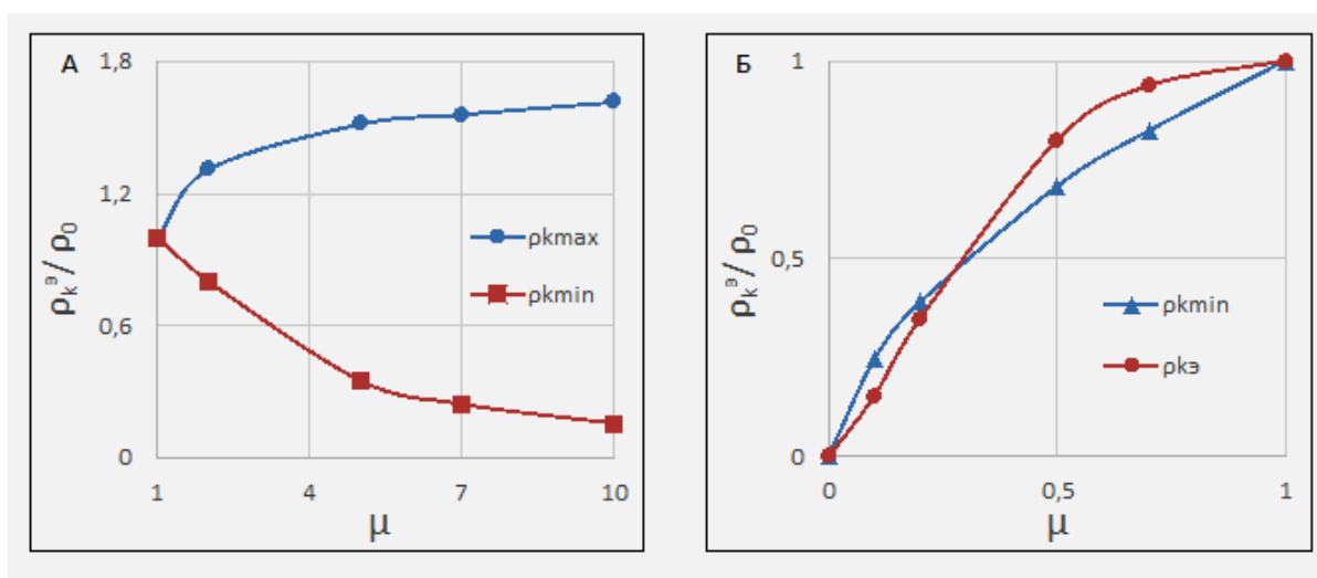
Рис. 5.6. Зависимости относительных значений УС ПЗ в точках экстремумов ( \rho_k^{\text{э}} / \rho_0 ) от параметра \mu = \rho^{\text{ист}} / \rho_0 для маломощного протяженного прослоя при h=0,5\text{AM}
