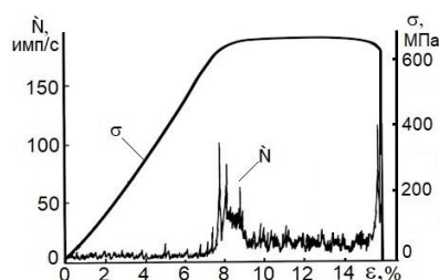
Рис.1. Зависимость активности АЭ \dot{N} и напряжения \sigma от степени деформации \varepsilon однослойного образца сплава П202.
