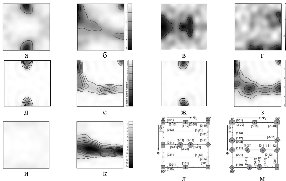
Рисунок 2. Эволюция кристаллографической текстуры IF-стали по промышленным переделам ее производства в виде сечений ФРО \varphi_2=0^\circ (а, в, д, ж, и) и \varphi_2=45^\circ (б, г, е, ж, з): а, б – ГП, центр; в, г – ГП, поверхность; д, е – ХП, центр; ж, з – ХП, поверхность; и, к – РО, вся толщина; л, м – шаблоны для расшифровки сечений ФРО с указанием вида с ПН основных ориентаций в виде элементарных ячеек ОЦК-решетки
