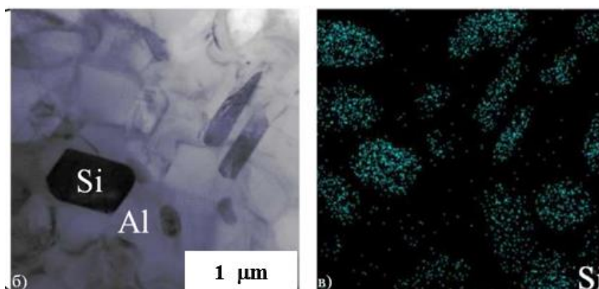
Рисунок 1. Экспериментальные изображения эвтектики алюминиево-кремниевого сплава, изготовленного аддитивным способом [5].
